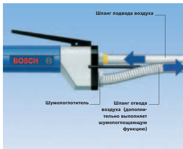
Рис. 7: Шланг отвода воздуха защищает пользователя, окружающую среду и обрабатываемую деталь
