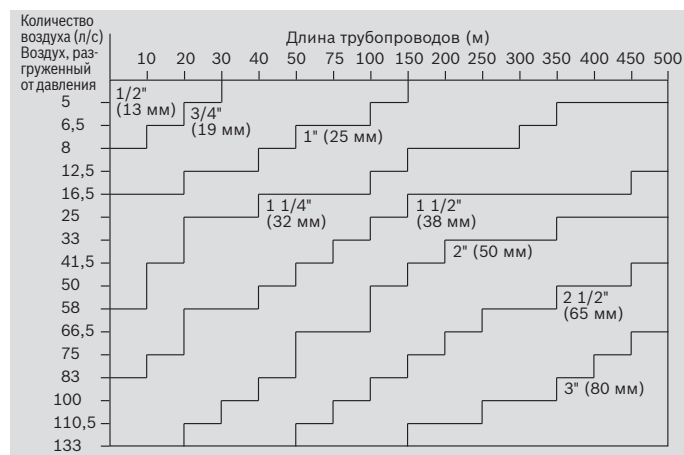
Рис. 5: Определение размеров трубопроводов
