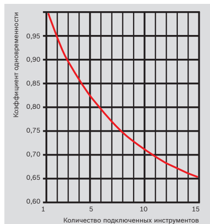
Рис. 3: Коэффициент одновременности
