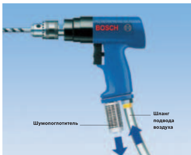
Рис. 6: Шумопоглотитель снижает до минимума уровень производственного шума
