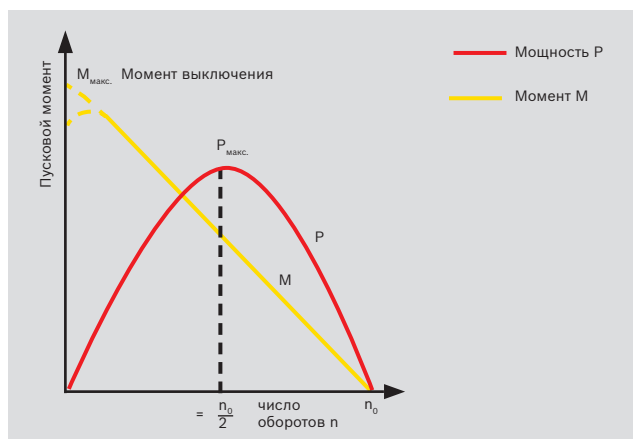
Рис. 1: Характеристики пневмодвигателя
